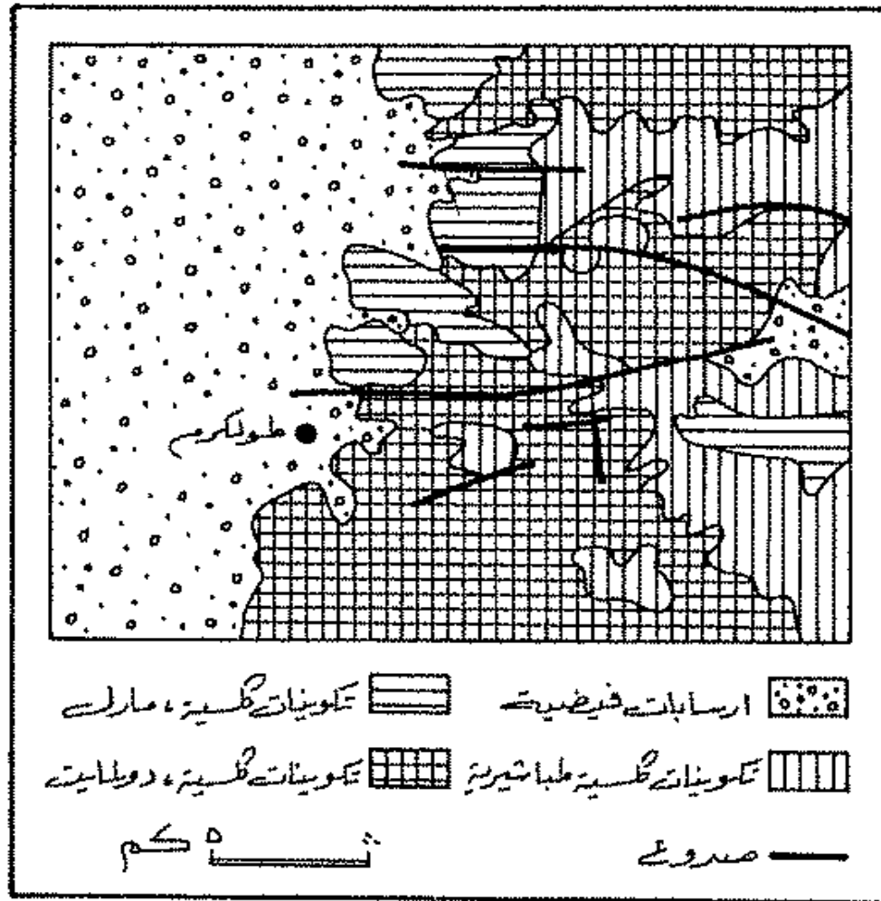
شكل (٣) التركيب الجيولوجي لمنطقة طولكرم
